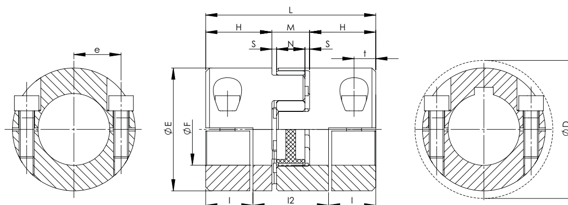
Figura 2-5 - TRASCO® ES - GESM
