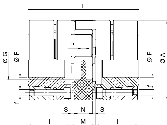
Figura 2-4 - TRASCO® ES esecuzione GESA
