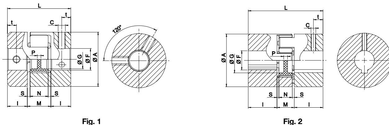
Figura 2-2 - Dimensioni TRASCO® ES: GESP e GESF
