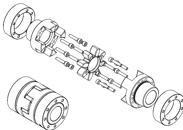
Figura 2-4 - TRASCO® ES esecuzione GESA
